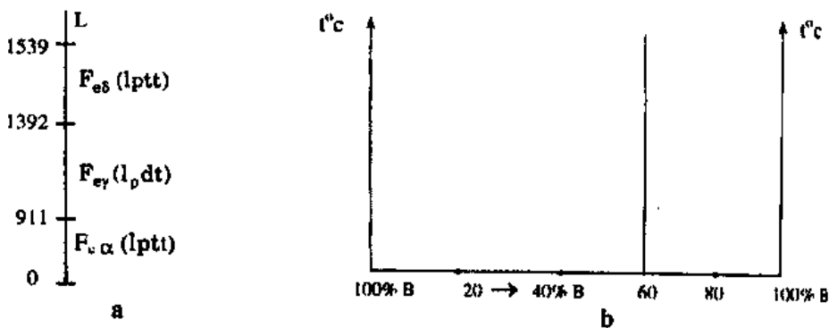
Hình 2.1 a) Giản đồ trạng thái một nguyên b) Giản đồ trạng thái hai nguyên
